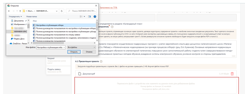
Рисунок 54. Диспетчер загрузки
