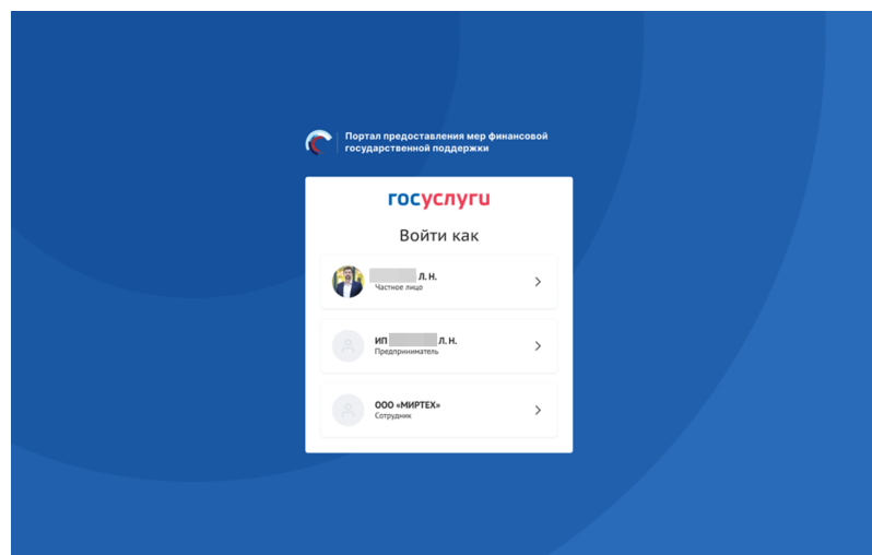
Рисунок 6. Выбор профиля
