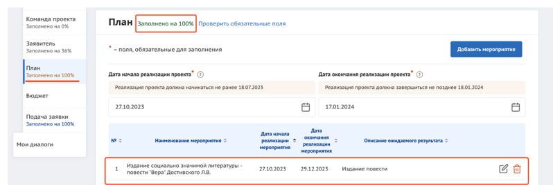
Рисунок 66. Таблица мероприятий
