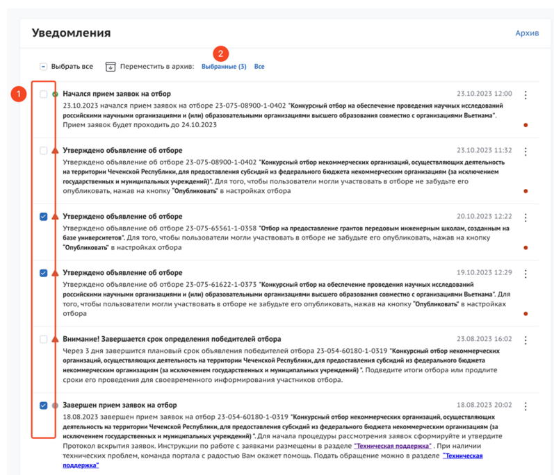
Рисунок 45. Множественный перевод
