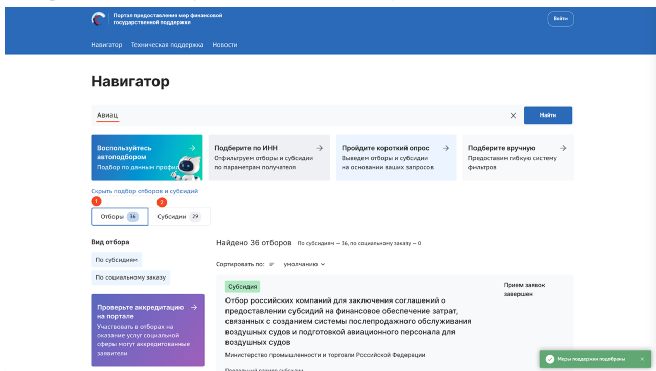
Рисунок 32. Страница «Навигатор»
