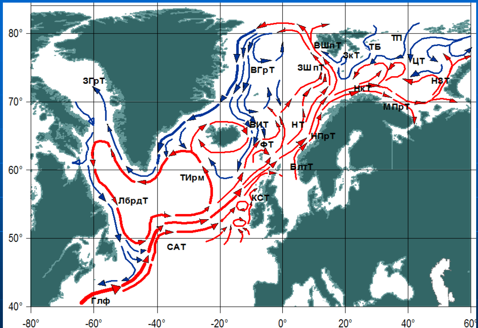
Генеральная схема поверхностных течений в Северной Атлантике, Норвежском, Гренландском и Баренцевом морях.
